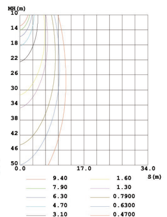
Iso-illuminance
